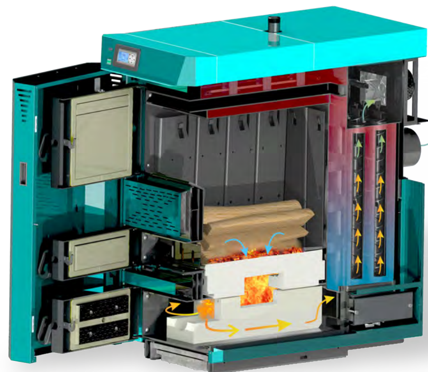
Presjek kotla
