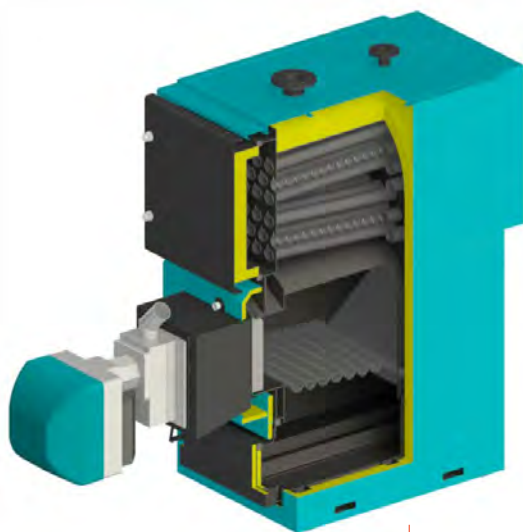
Presjek kotla
