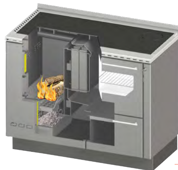
Presjek kotla
