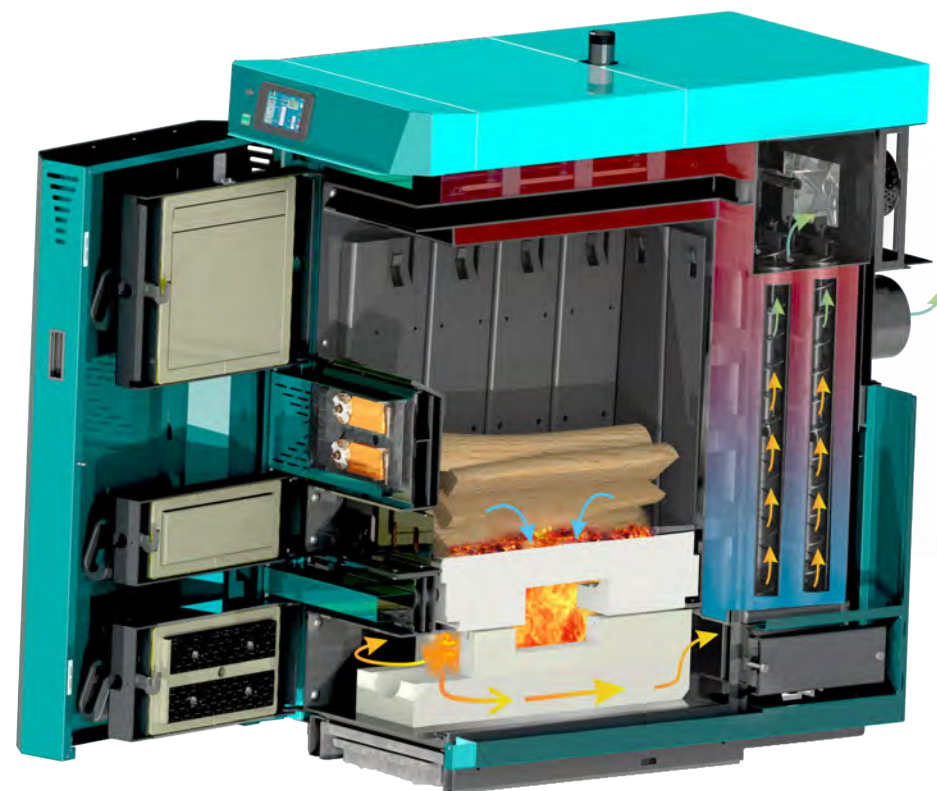
Presjek kotla
