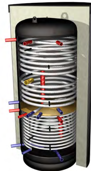
Presjek spremnika
